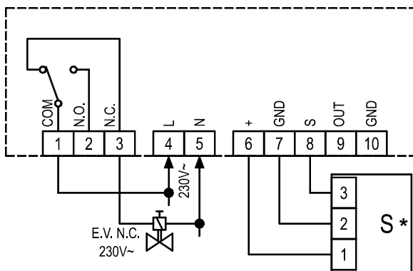
Fig. 8: Esquema de ligação com electroválvula com rearmação manual, normalmente fechada a 230V~, com sensor remoto * (cód.: SGA---).
